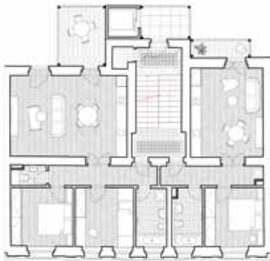
Půdorys 2. NP
